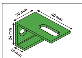
Art. K075/2 ülemine siin (alumiinium)
