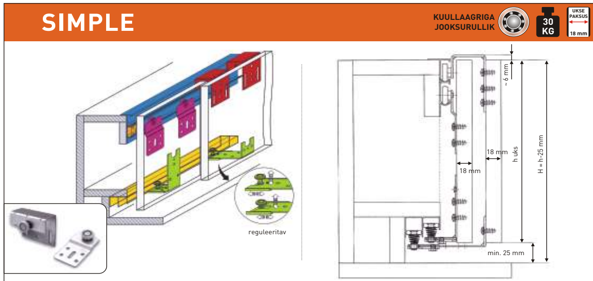
Art. 3328 kinnituste komplekt (2 ust)
