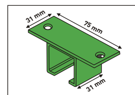
Art. 1132 topelt laekinnitus
