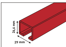
Art. K075/3,5 ülemine siin (alumiinium)
